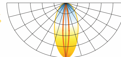
ГРАФИК РАСПРЕДЕЛЕНИЯ СВЕТА Угол рассеивания 10x65°
