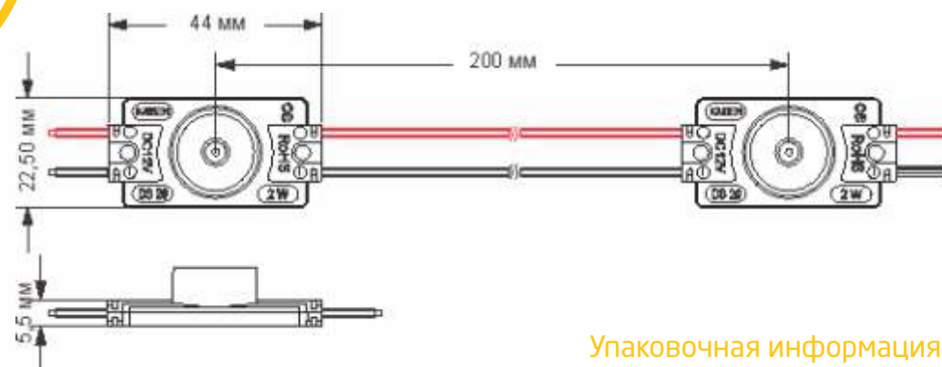
РАЗМЕРЫ
