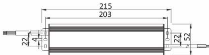
ГАБАРИТНЫЕ РАЗМЕРЫ
