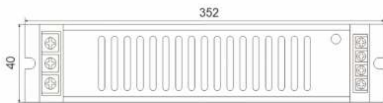
ГАБАРИТНЫЕ РАЗМЕРЫ
